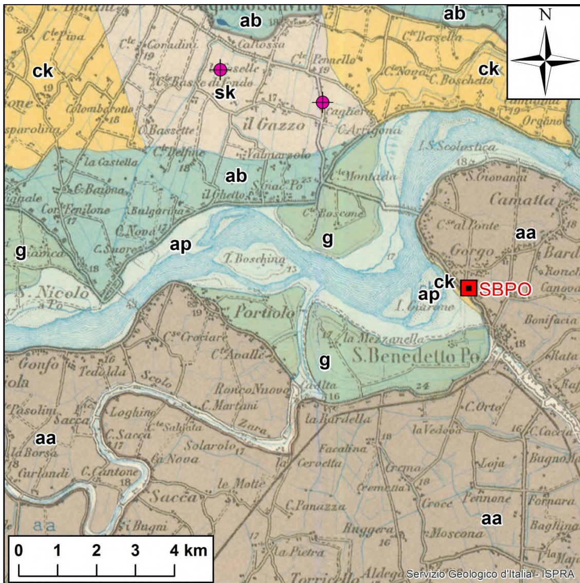
Stralcio del Foglio 62 Mantova della Carta Geologica d'Italia in scala 1:100.000 con l'ubicazione della Stazione Sismica e di due sondaggi di riferimento dell'Archivio ex L464/84 ISPRA (cerchi viola).
