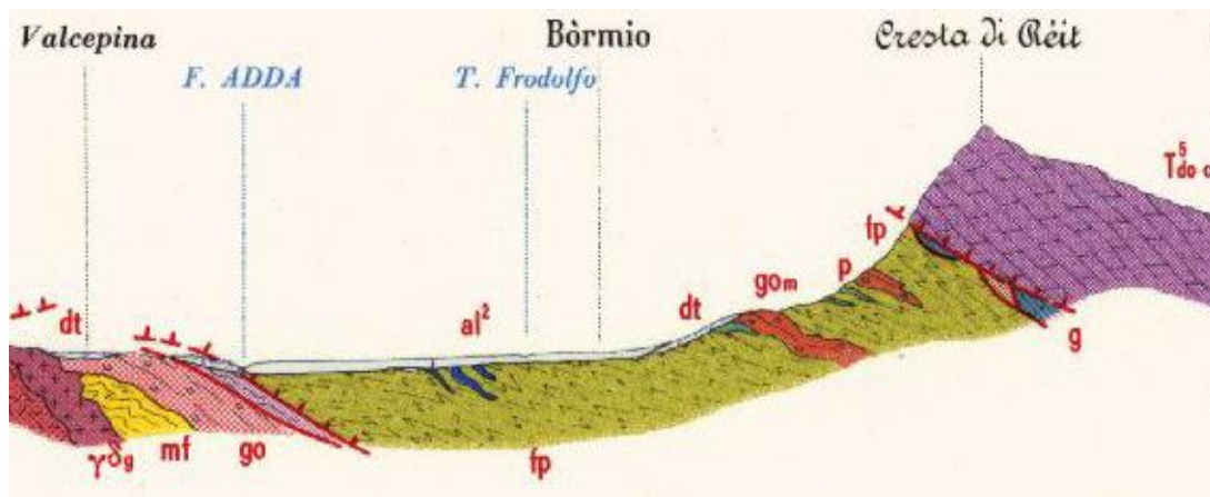
Stralcio della Sezione geologica III (direzione SSW-NNE) del Foglio 8 Bormio della Carta Geologica d'Italia scala 1:100.000 nel tratto in corrispondenza della stazione sismica.
