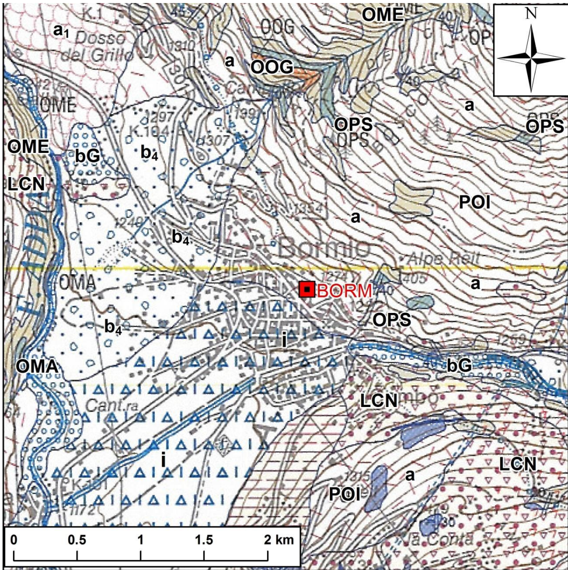
Stralcio del Foglio 024 Bormio della Carta Geologica d'Italia scala 1:50.000 (ingrandito in scala 1:30.000) con l'ubicazione della Stazione Sismica.
